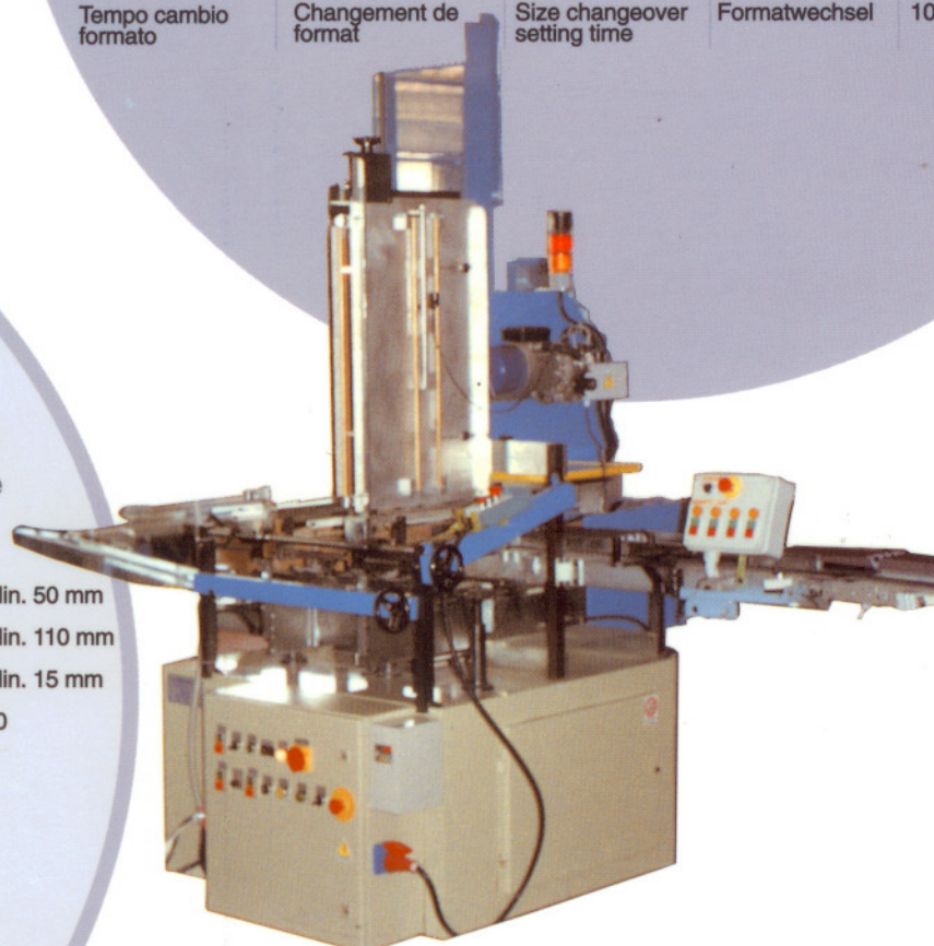
5. EPC170 Tappatrice Fermeuse de boîtes Box/Lid closer Schachtel Verschlussmaschine
